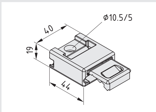
Zahnriemenspanner Spannblock 8 R25, 0.0.426.29 [b]
