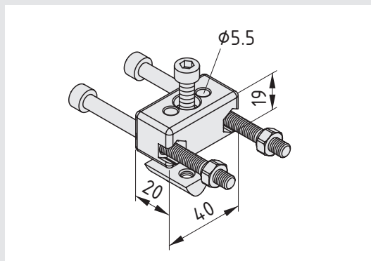
Zahnriemenspanner Gegenlager 8 R25, 0.0.426.30 [a]
